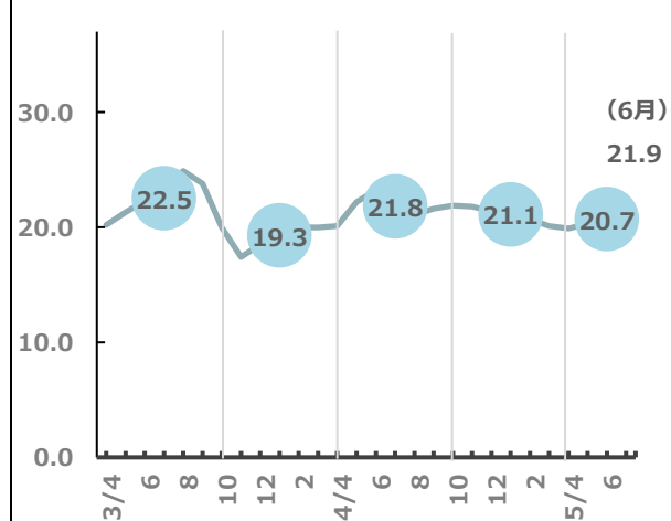
Mo($/lb)
