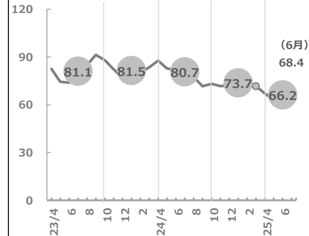
原油ﾄﾞﾊﾞｲ($/B)
