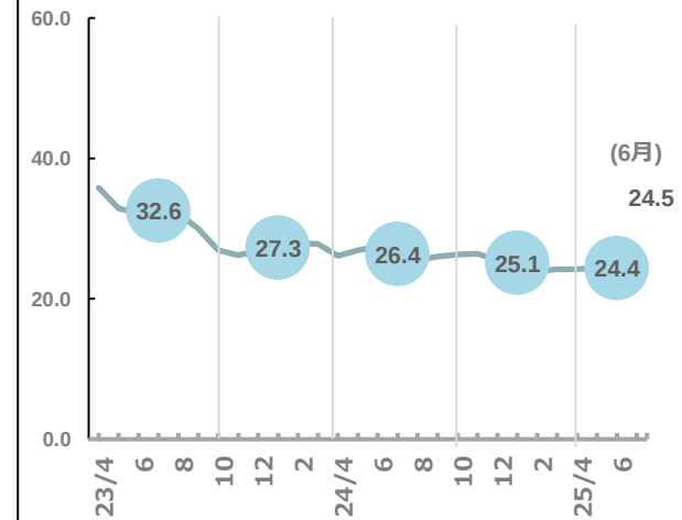
V($/Kg)
